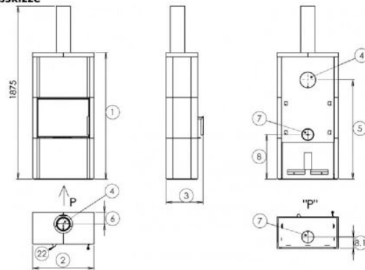
Maßskizze
