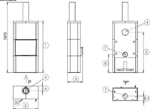
Maßskizze
